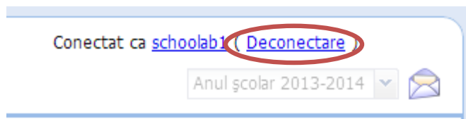
Figura 12. Buton „Deconectare”
