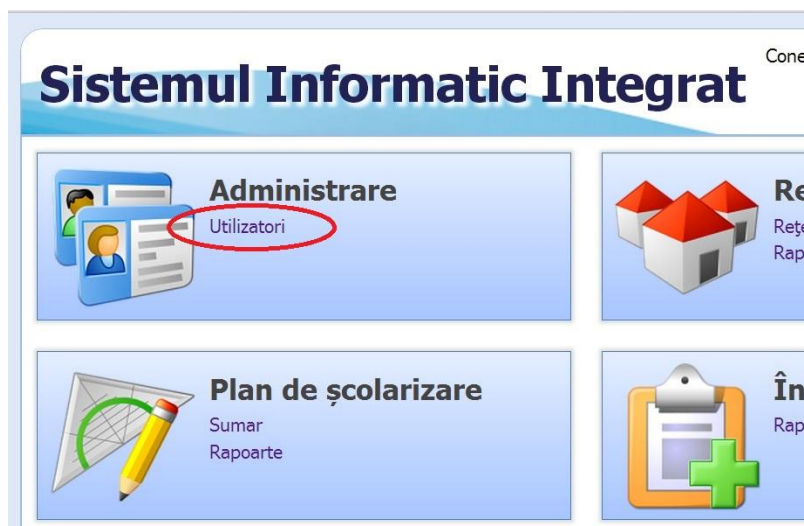
Figura 7. Modul Administrare
